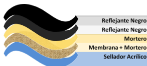
Imperlasa i7
